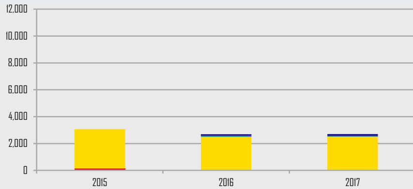
CO 2 -Emissionen insgesamt (in Tonnen CO 2 )
