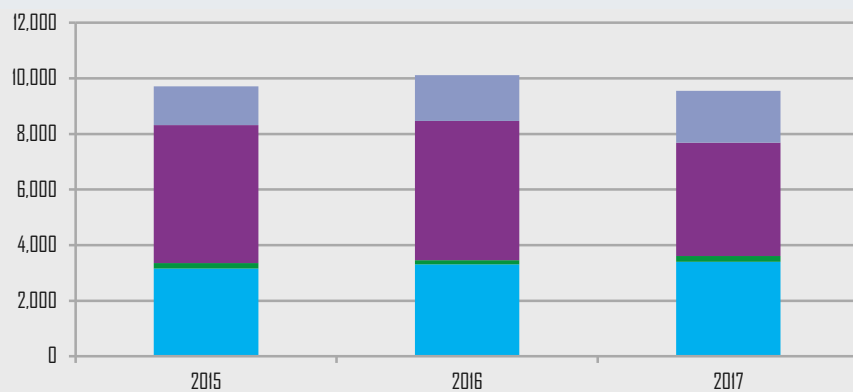
CO 2 -Emissionen insgesamt (in Tonnen CO 2 )
